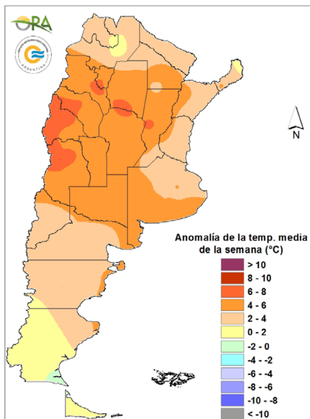
Anomalia de la temperatura media de la semana del 19/02/2025 al 25/02/2025
