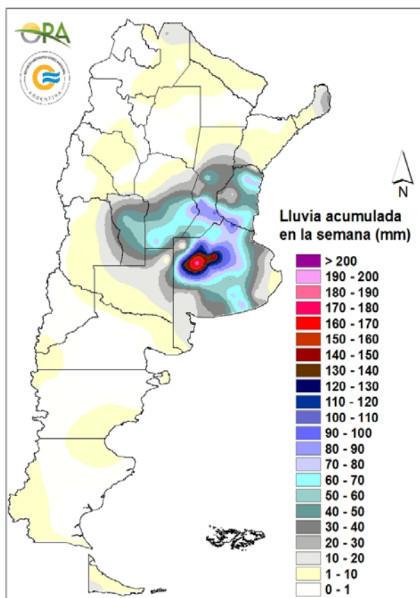
Precipitaciones acumuladas en la semana del 19/02/2025 al 25/02/2025
